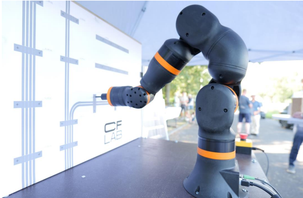
↗ Großraummanipulatoren
